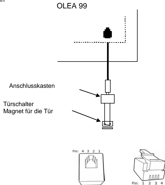
Abbildung 5 Pin – Reihenfolge von RJ 10
