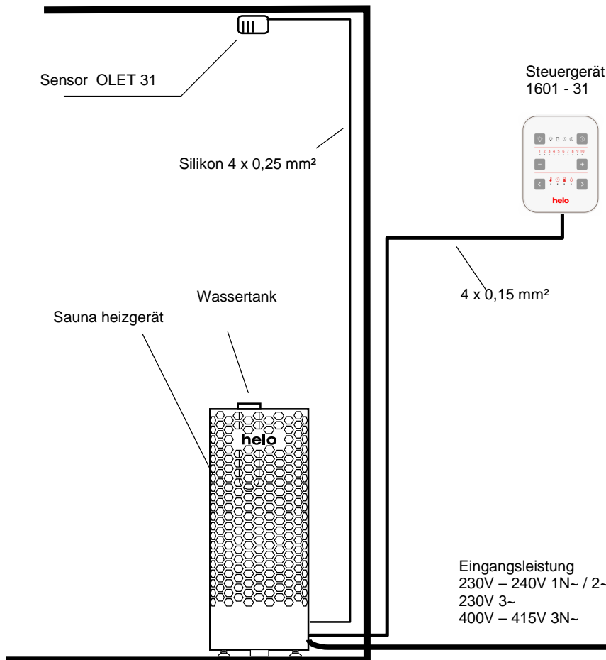
Abbildung 8 Prinzipbild
