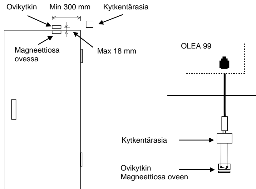
Kuva 4 Ovikytkimen asento
