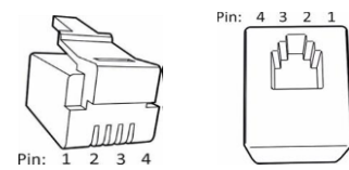
Kuva 5. RJ 10 liittimen Pin -järjestys
