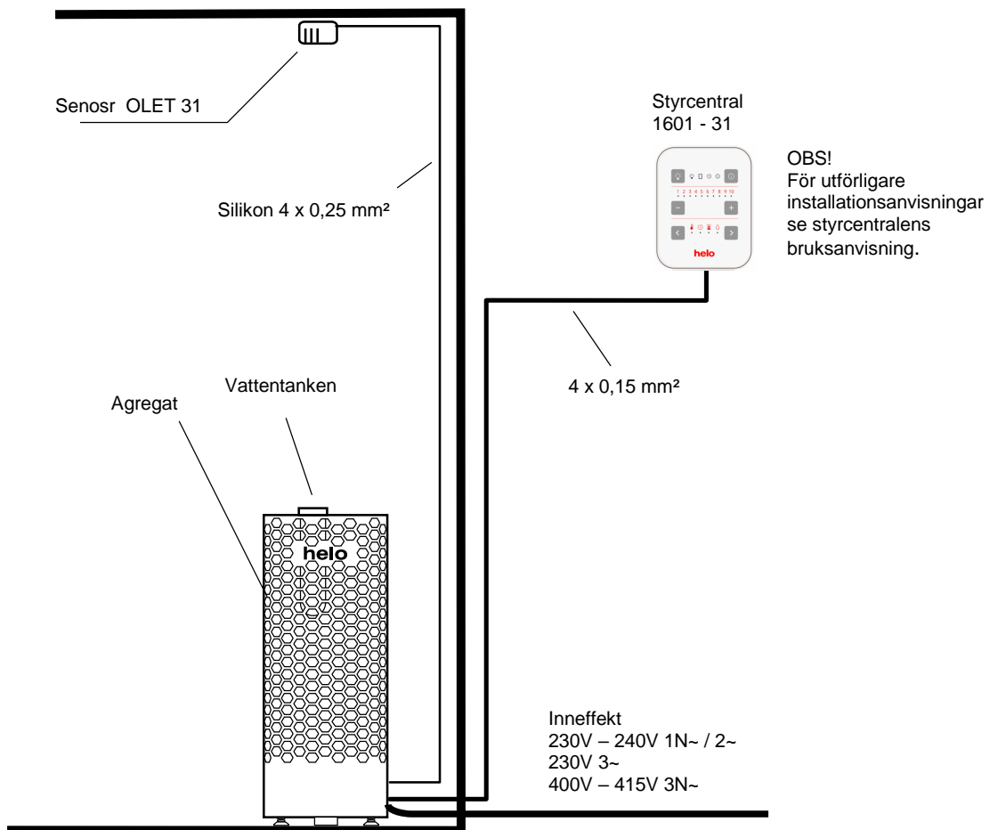
Bild 8 Principskiss
