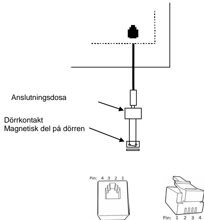
Bild 5 Stift-order av RJ 10
