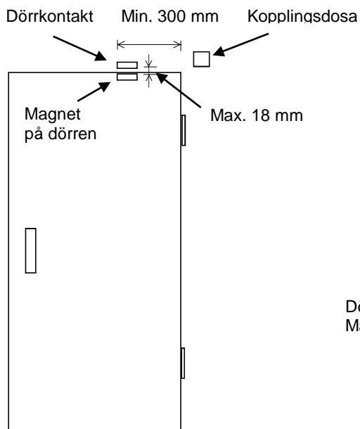
Bild 4 Montering av dörrkontakten
