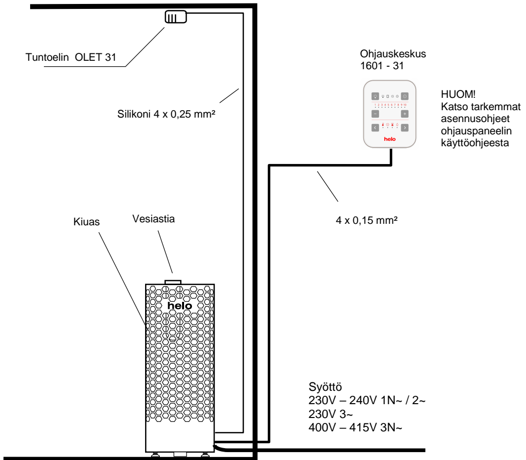
Kuva 8 Periaatekuva kytkennästä
